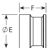
Montagekupplung
